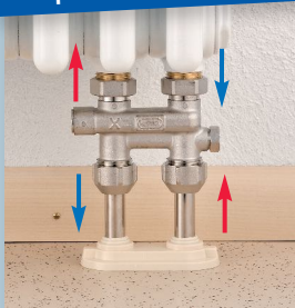
Ravni H-ventil X razdjelnik s ravnim priključkom s mogućnošću zatvaranja za 1 i 2 - cjevne sustave grijanja
